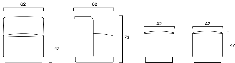
Clubby Dining FG49301 / 49331 / 49321 / 49341 / 49351 / 49361
